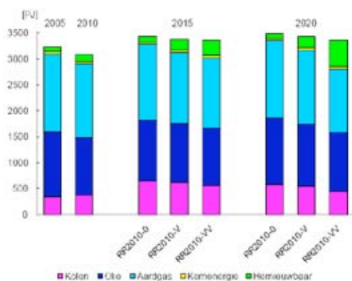
Figuur 1: Energiemix 2005-2020 41)
